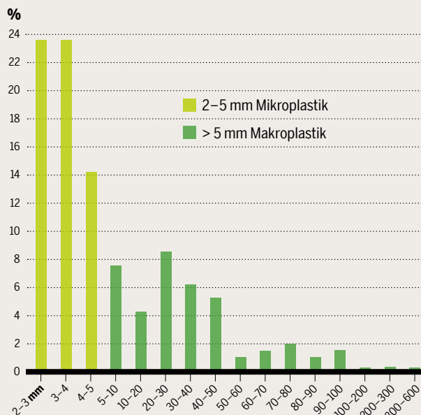
Größenspektrum der Plastikpartikel im Boden in Millimeter, Verteilung in Prozent
